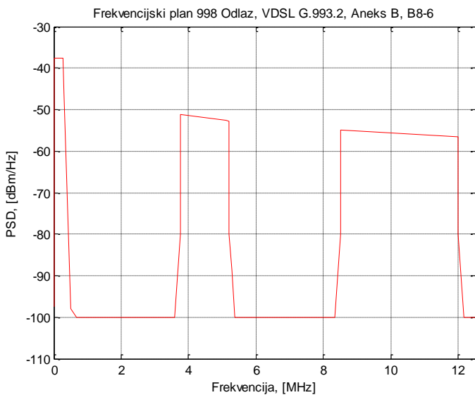
Slika 5.7.2 5.7.2 Frekvenijski predložak za odlazni smjer prijenosa za VDSL2, frekvenijski plan 998, B8-6
