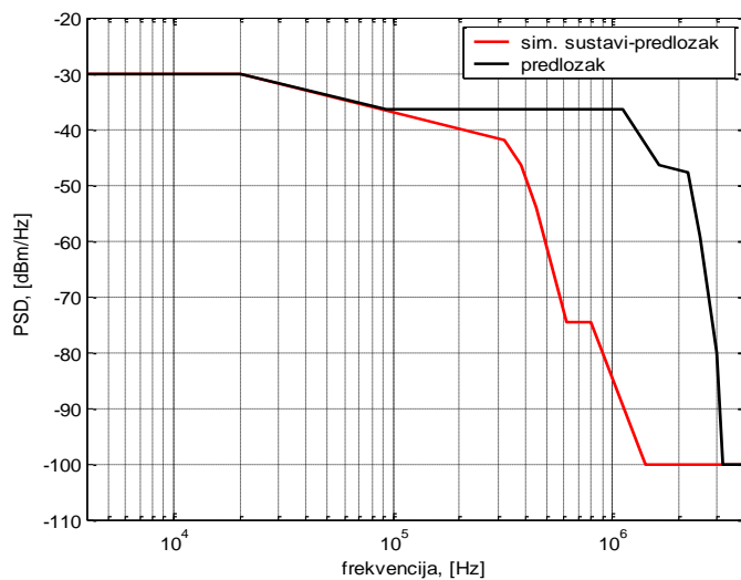
Slika 5.2.1 Frekvenijski predložak za asimetrične sustave prijenosa (dolazni smjer)
