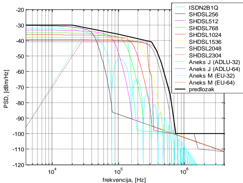
Slika 5.7.5 Frekvenijski predložak za odlazni smjer prijenosa (pretplatničke linije srednje duljine).
