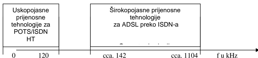
Slika 1. Frekventijski opseg za uskopojasne i širokopojasne prijenosne tehnologije
