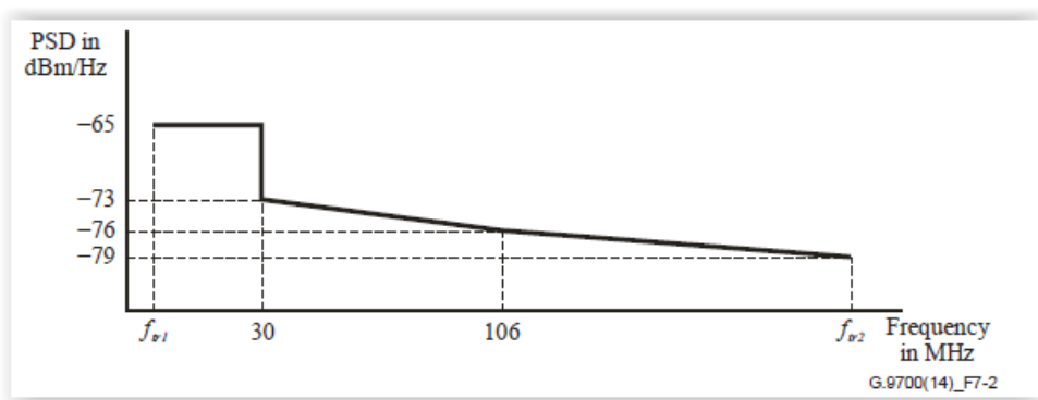
Slika 4.9.2 - Maska PSD za G.Fast 212 MHz profil
