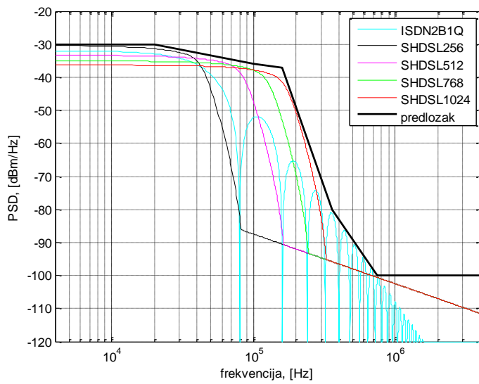
Slika 5.7.7 Frekvencijski predložak za odlazni smjer prijena (duge pretplatničke linije) za ADSL preko POTS (aneks A).
