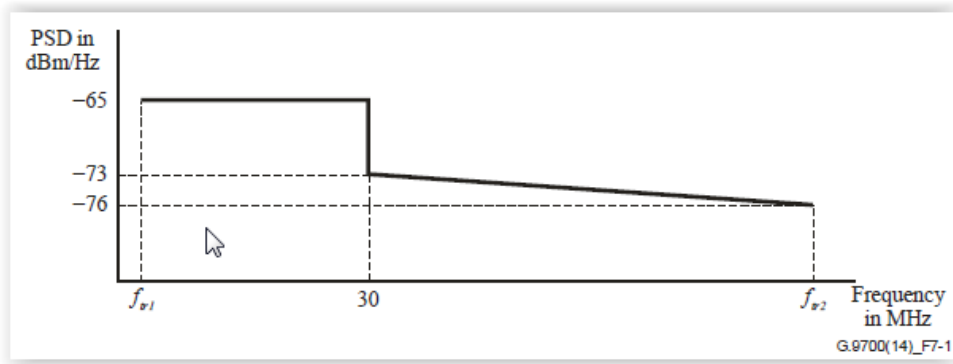
Slika 4.9.1 - Maska PSD za G.Fast 106 MHz profil
