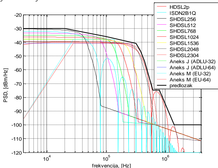
Slika 5.7.1 Frekvencijski predložak za odlazni smjer prijensa (kratke pretplatničke linije).
